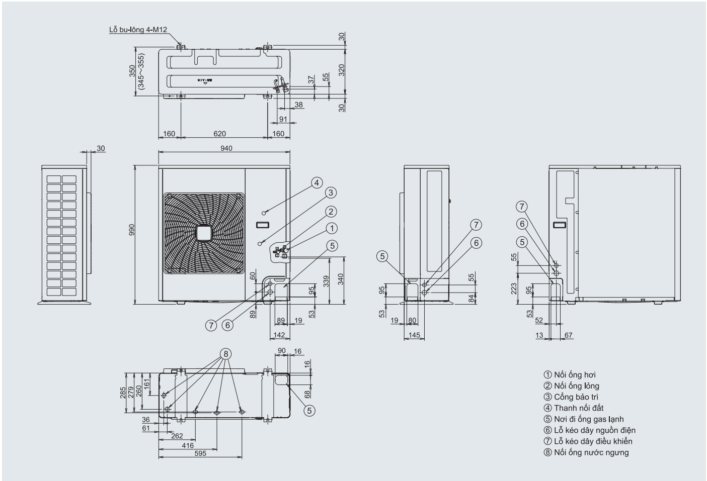
DÀN NÓNG // RNQ36MV1V
