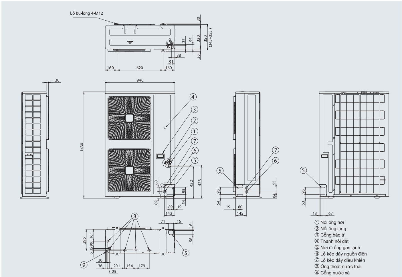
DÀN NÓNG // RNQ36MV1V
